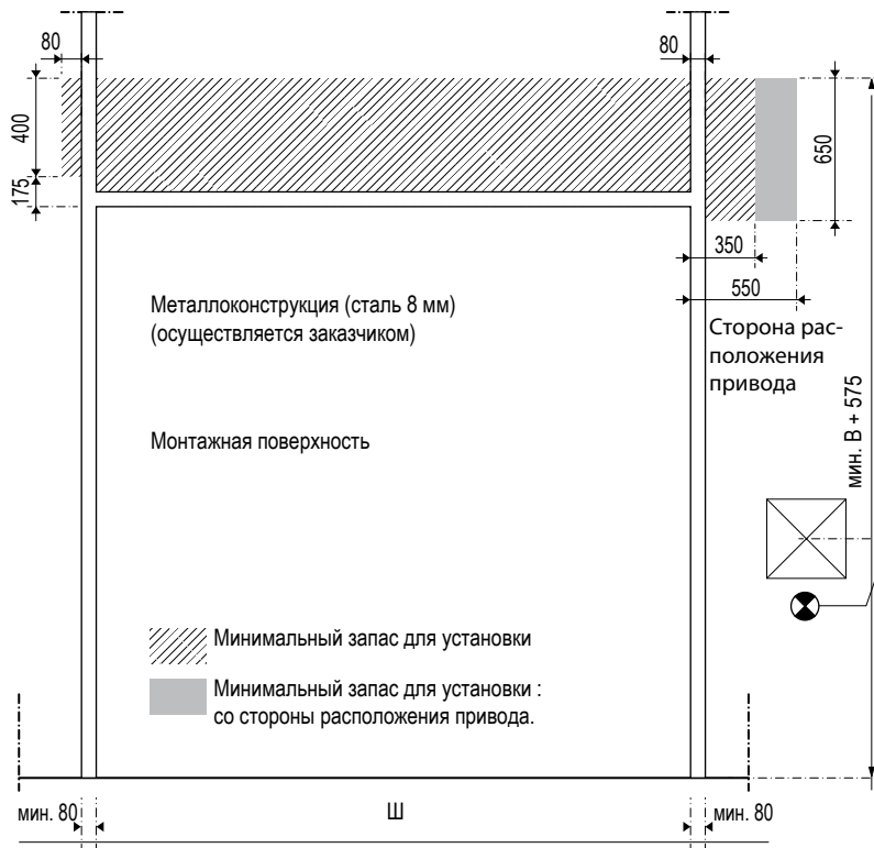
Разрез А
